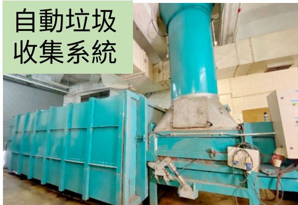
吸管將投入每層垃圾槽口的垃圾輸送到地下垃圾站，經壓縮後再運走
